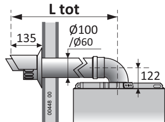
Ejemplo de sistema coaxial horizontal ( C_{13} )
